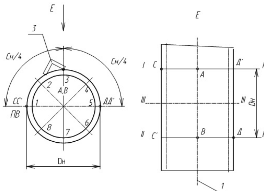
ЛЕКАЛО ОВАЛА
