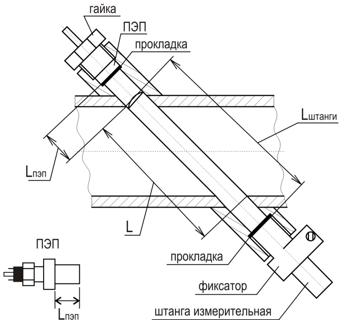
Измерение расстояния между ЦЭП в УПР
