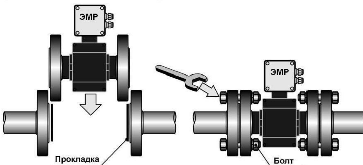
Рисунок 6.4 - Способ установки расходомеров
