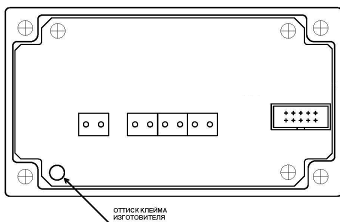
Рисунок 4.3 – Места пломбирования
