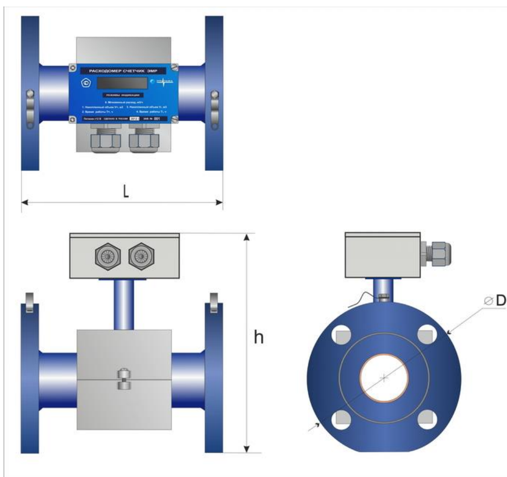
Рисунок 2.1 - Габаритные и установочные размеры расходомеров.
