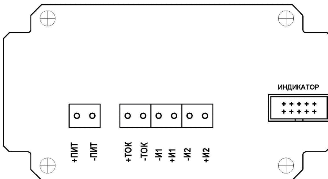
Рисунок 4.1 – Внешний вид платы
