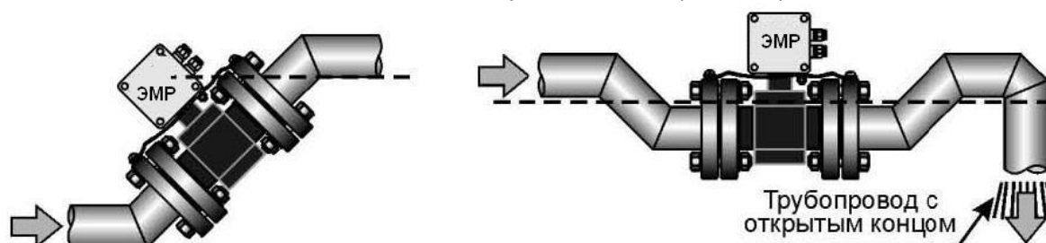
Рисунок 6.2 - Установка ЭМР при измерении расхода в частично заполненном трубопроводе
