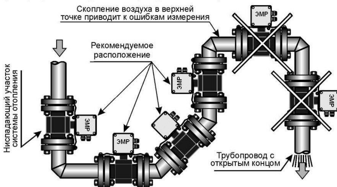
Рисунок 6.1 - Пример установки расходомеров
