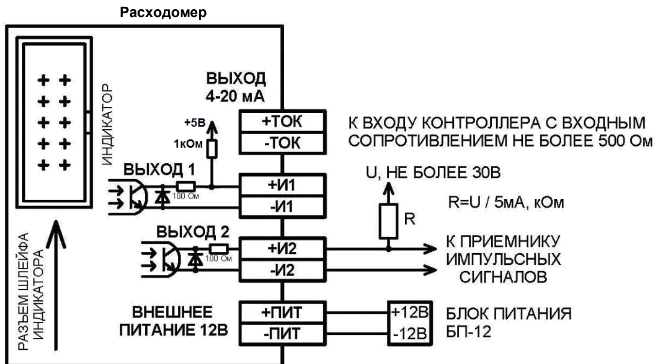
Рисунок 4.2 – Подключение к ЭМР
