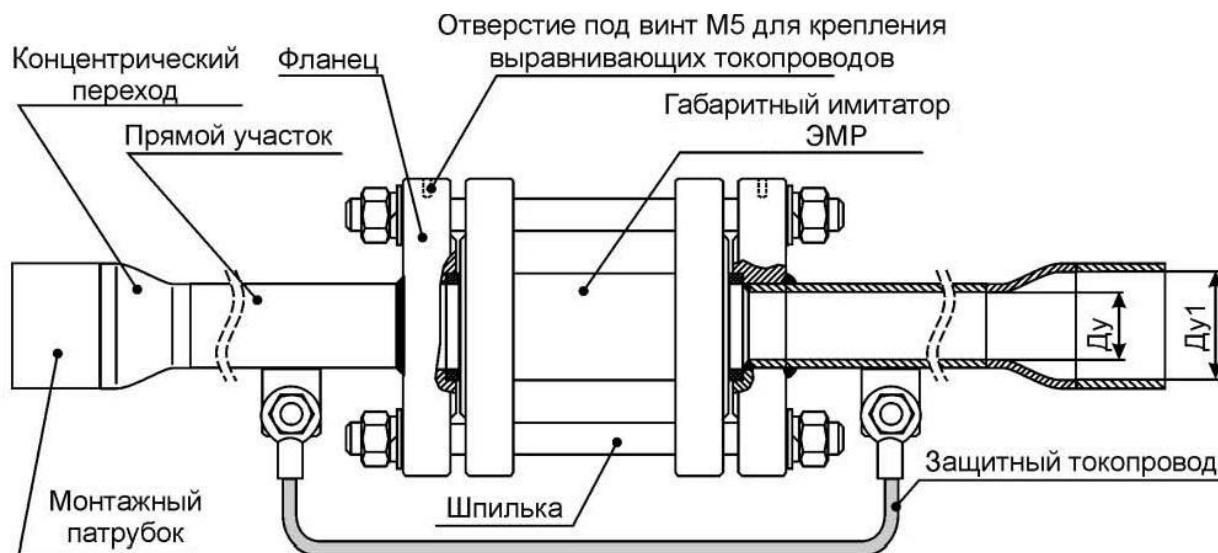
Рисунок 6.6 Внешний вид КМ
