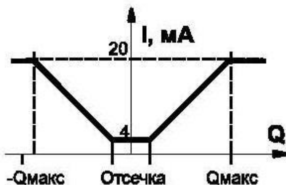
Рисунок 4.5 - Выходная характеристика токового выхода
